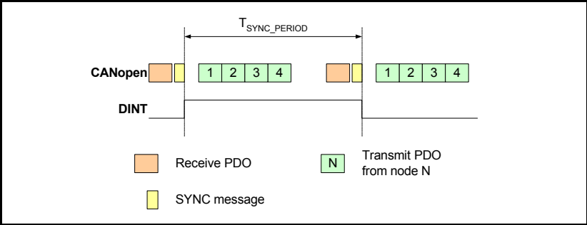
Figure 11-11 DINT
